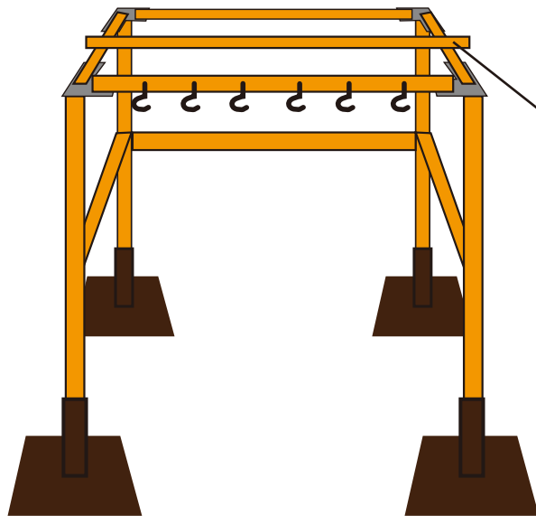
⑤よしず受けの棒をのせます。 凹を横棒にはめ込み固定します。
